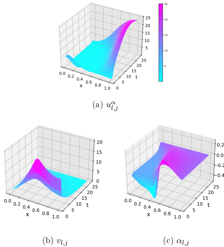
Рис. 3. Графики (а) распределения пользователей по степени вовлеченности u_{l,j}^\alpha модели с уравнением типа КФП (3), (б) функции стоимости v_{l,j} модели с уравнением типа ГЯБ (5), l = 0, \dots, N_t , j = -1/2, \dots, N_x + 1/2 и (с) функции управления \alpha_{l,j} , удовлетворяющей условию оптимальности (6), l = 0, \dots, N_t , j = 0, \dots, N_x .
