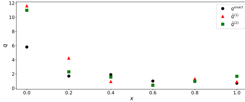
Рис. 6. Восстановленные значения вектора параметров q \in \mathbb{R}^6 . Черные точки — точные значения параметров обратной задачи q^{exact} , красные треугольники — восстановленные значения параметров \hat{q}^{(1)} обратной задачи 1, зеленые квадраты — восстановленные значения параметров \hat{q}^{(2)} обратной задачи 2.
