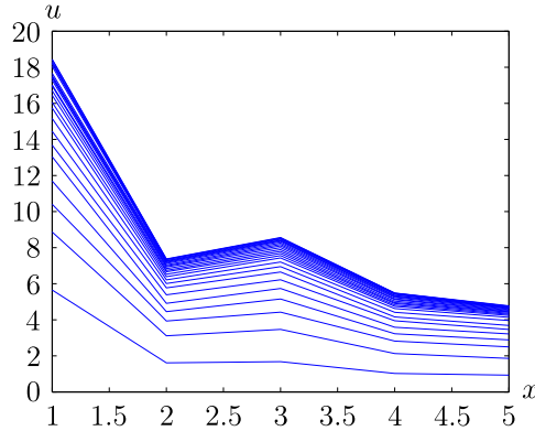
Рис. 1. Данные новостного сайта Digg.com (плотность вовлеченных пользователей за 50 часов) [6].
