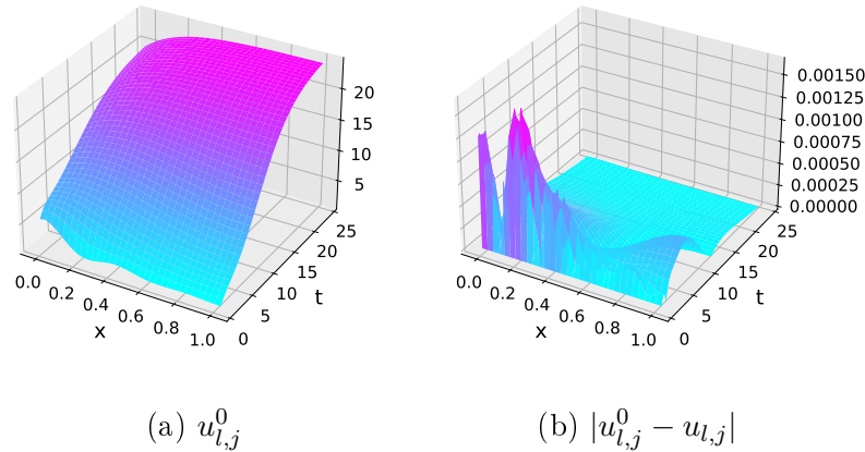
Рис. 2. Графики (a) распределения пользователей по степени вовлеченности u_{l,j}^0 модели с уравнением типа КФП (3) при \alpha = 0 и (b) абсолютной разности |u_{l,j}^0 - u_{l,j}| , l = 0, \dots, N_t, j = -1/2, \dots, N_x + 1/2 .
