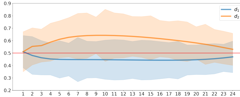
Рис. 4. Графики значений глобальных индексов чувствительности S_m , m = 1, 2 для коэффициентов d_1 и d_2 функционала стоимости (2) для t = 1, \dots, 24 . Полупрозрачные полосы — 95% доверительные интервалы.
